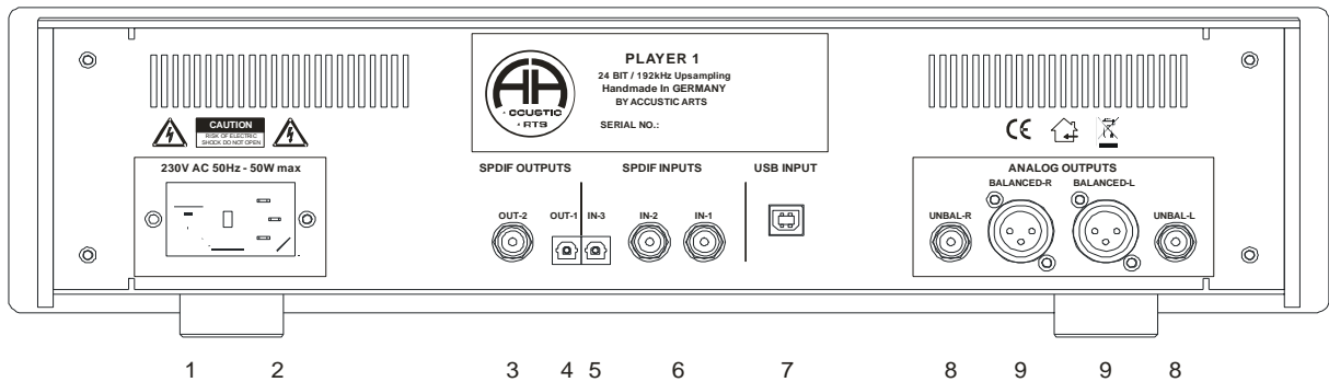
Grafik 1: Rückansicht
