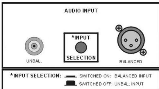
Grafik 2: Eingangsumschaltung INPUT SELECTION
