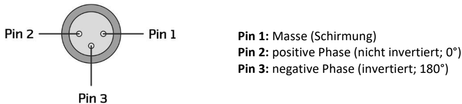
Grafik 3: Pin-Belegung eines symmetrischen Eingangs (XLR)
