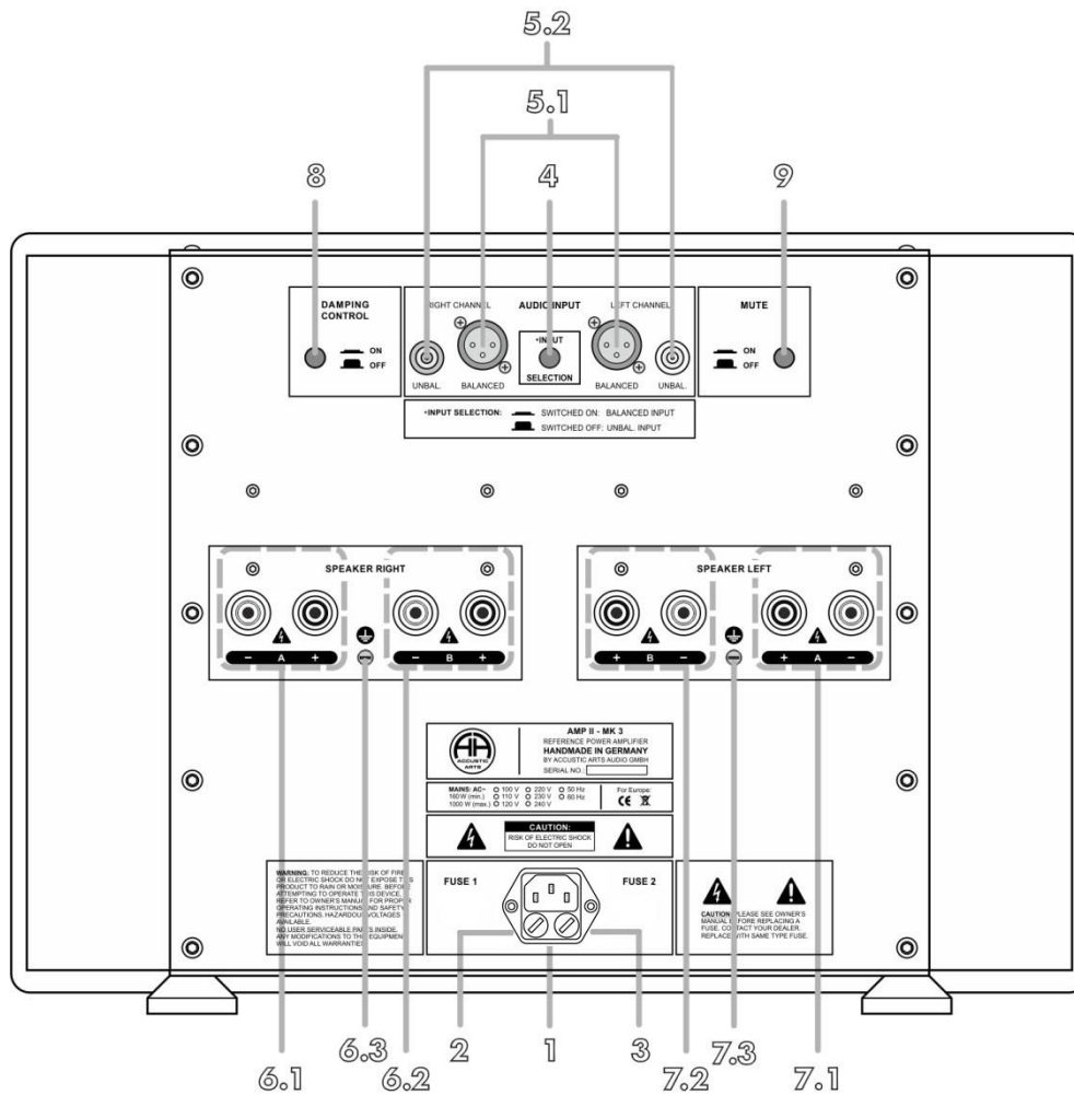
Grafik 1: Rückansicht
