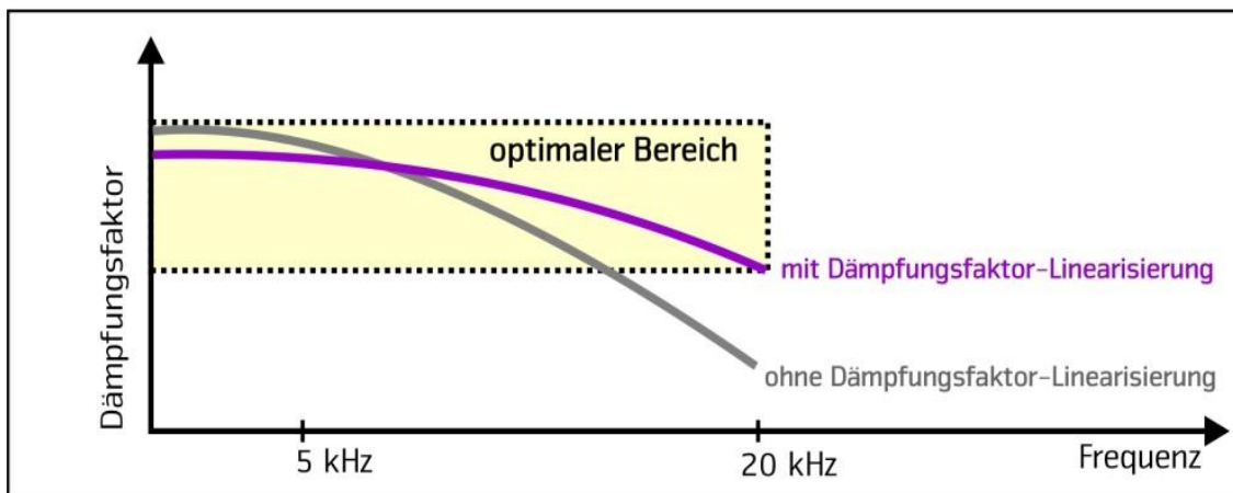
Grafik 5: Stark vereinfachtes Diagramm zur Veranschaulichung der Dämpfungsfaktor-Linearisierung
