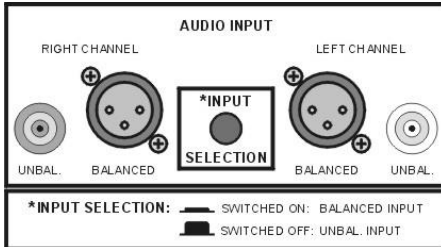
Grafik 2: Eingangsumschaltung INPUT SELECTION
