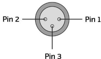
Grafik 3: Pin-Belegung eines symmetrischen Eingangs (XLR)
